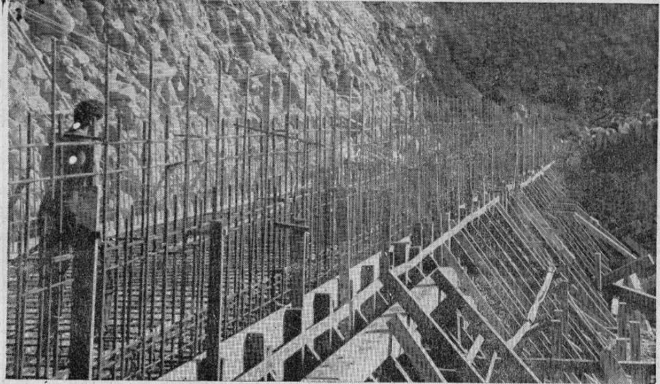
Preparación de la armadura para la chorroa del Canal Lateral del desarenador de La Planta Hidroeléctrica de LA GARITA.
